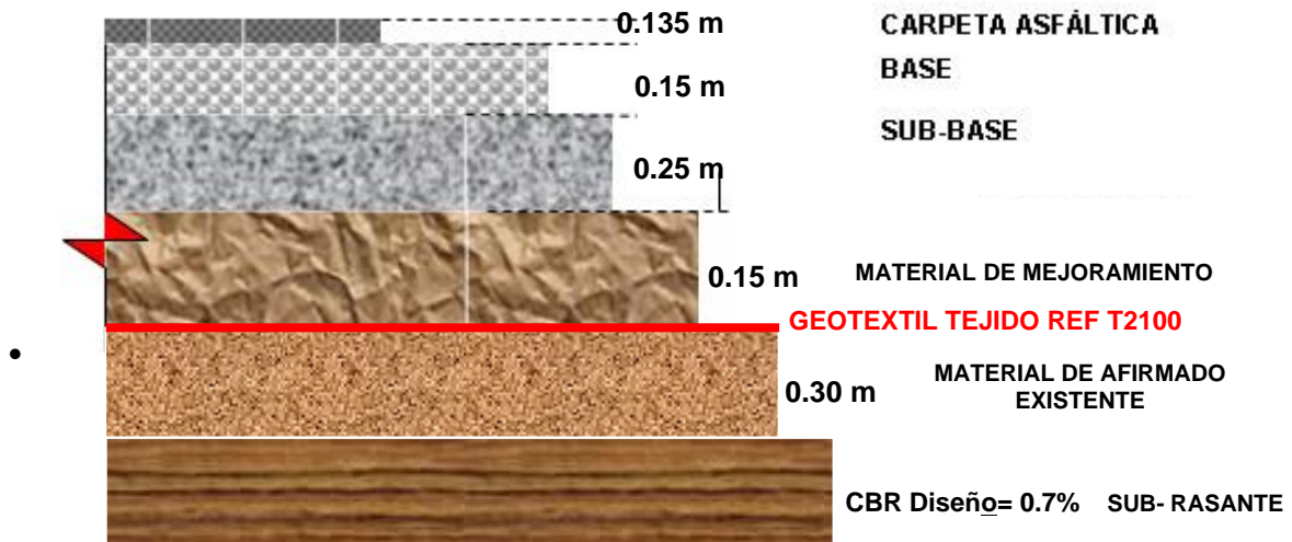
Ilustración 20 Dimensionamiento de la estructura en pavimento flexible para la zona particular N°1 de la unidad de diseño N°2 del tramo N°1- Fuente: El Autor
