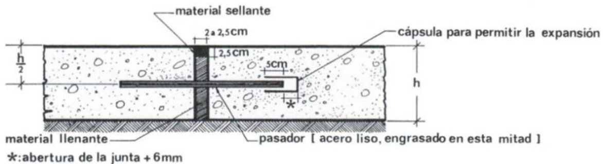
Ilustración 12 Junta de expansión con dovela tipo 1
