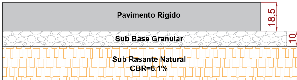
Ilustración 5 Dimensionamiento de la estructura de pavimento rigido para la unidad de diseño N°1 del tramo N°1 (Dimensiones en cm)- Fuente El Autor
