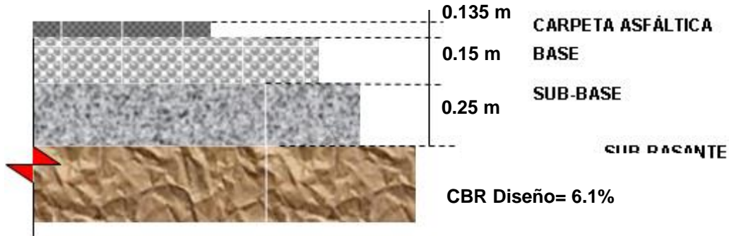
Ilustración 19 Dimensionamiento de la estructura en pavimento flexible para la unidad de diseño N°2 del tramo N°1
