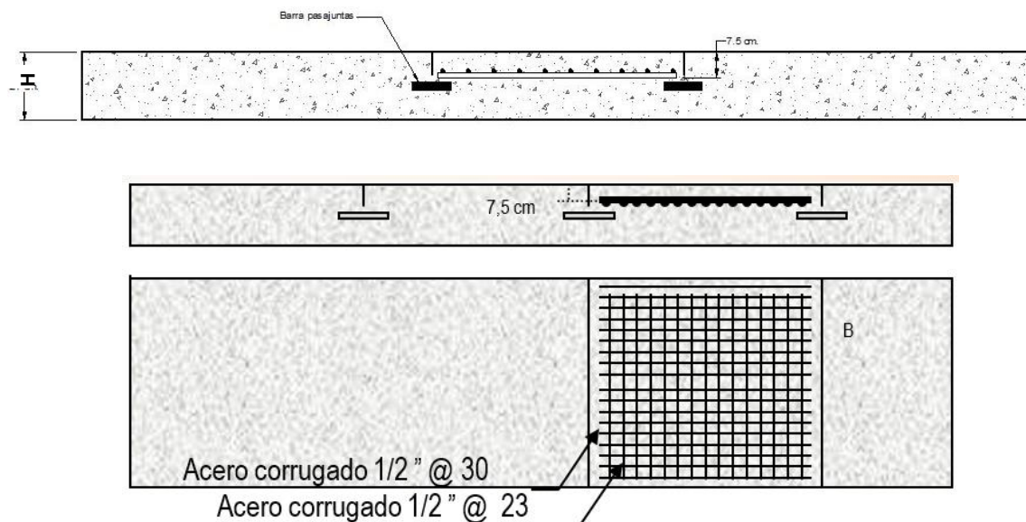
Ilustración 14 Disposición típica de acero de refuerzo en casos especiales
