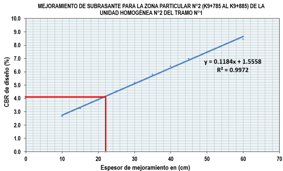
Grafica 2 Determinación del espesor de mejoramiento para la obtención de un CBR de diseño igual o mayor a 10% para la zona particular N°2 de la unidad de diseño N°2 del tramo N°1- Fuente: Elaboración propia
