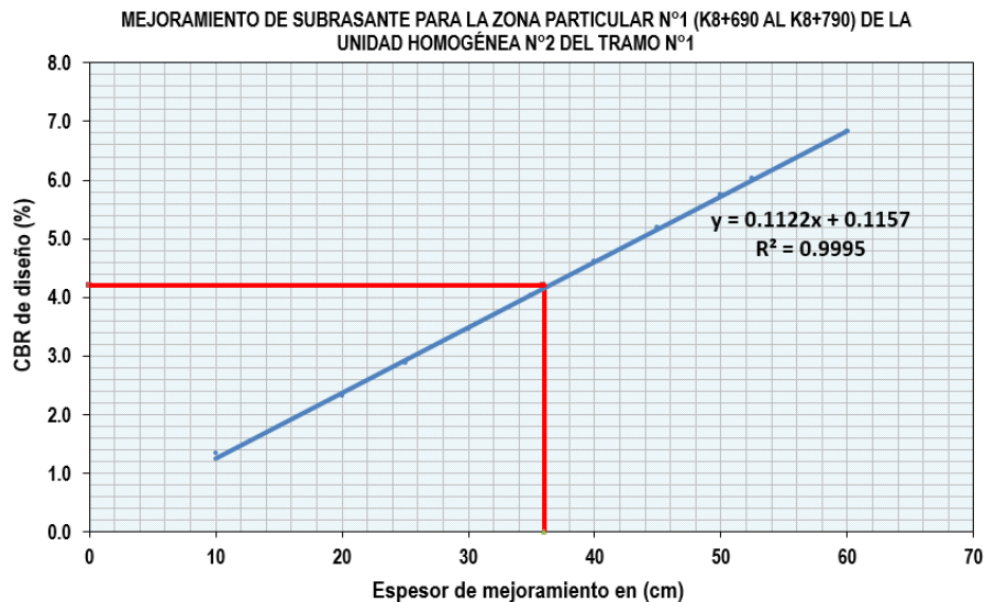
Grafica 1 Determinación del espesor de mejoramiento para la obtención de un CBR de diseño igual o mayor a 10% para la zona particular N°1 de la unidad de diseño N°2 del tramo N°1- Fuente: Elaboración propia
