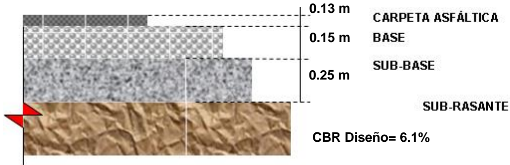
Ilustración 18 Dimensionamiento de la estructura en pavimento flexible para la unidad de diseño N°1 del tramo N°1
