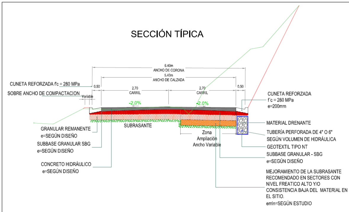
Figura 2 Sección Transversal Tipo a implementar
