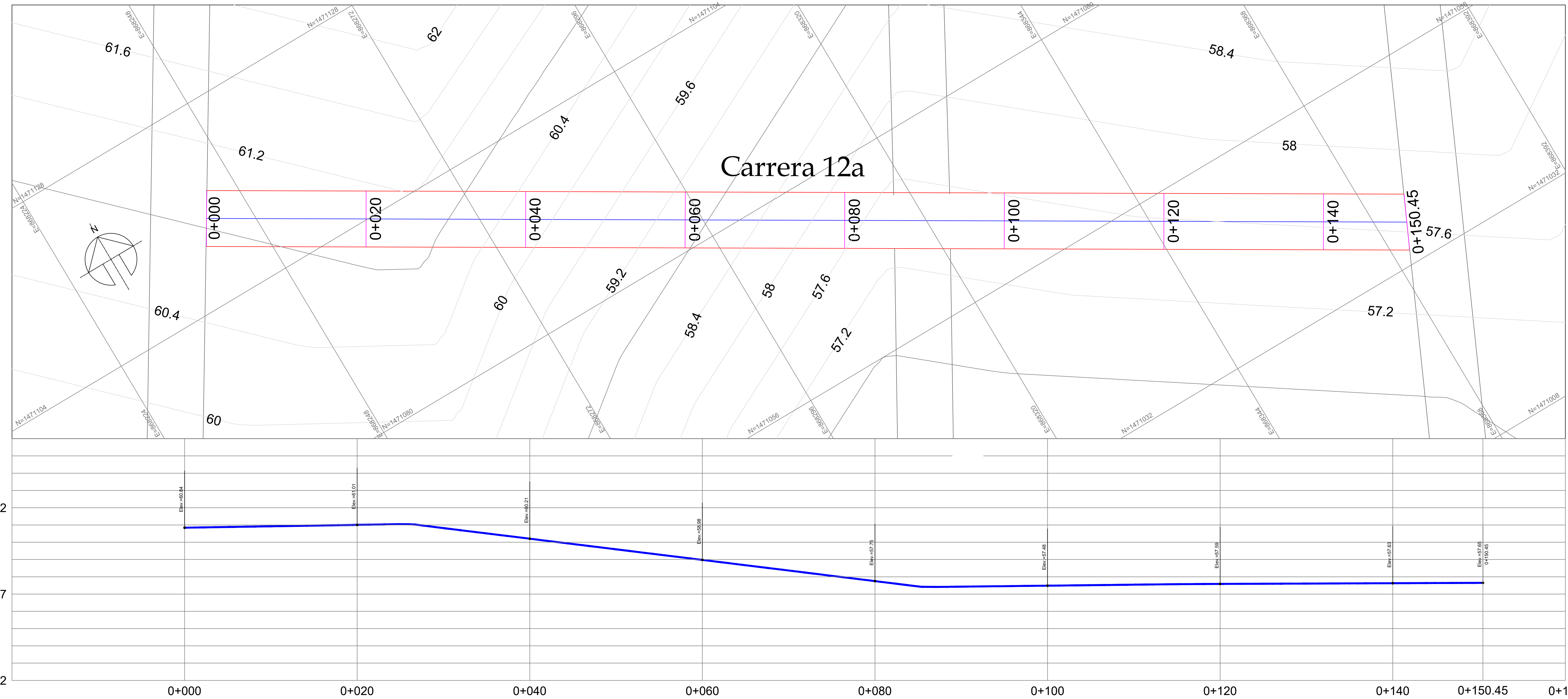
PERFIL ESCALA HORIZONTAL 1:100 ESCALA VERTICAL 1:50
