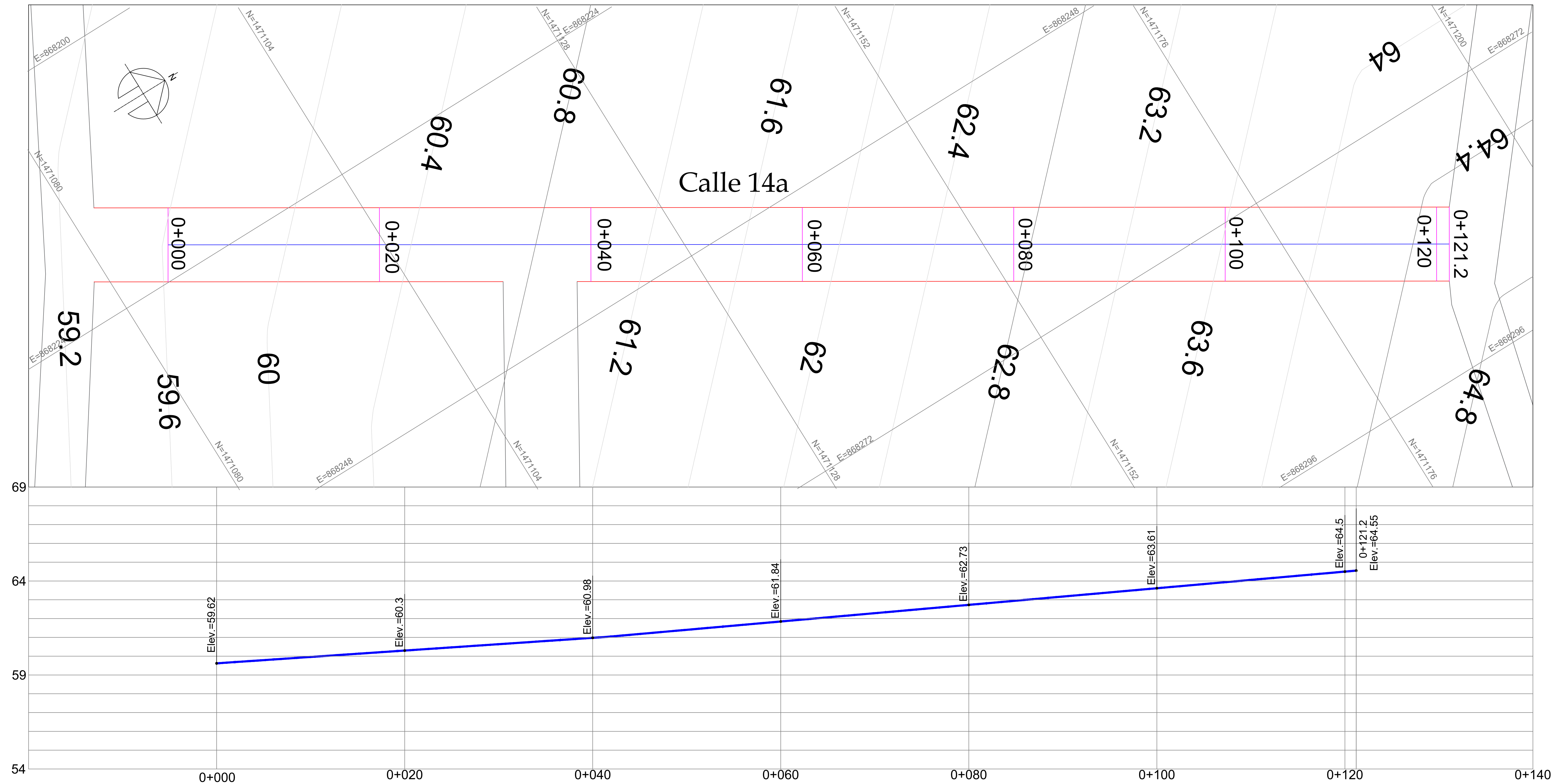
PERFIL ESCALA HORIZONTAL 1:100 ESCALA VERTICAL 1:50
