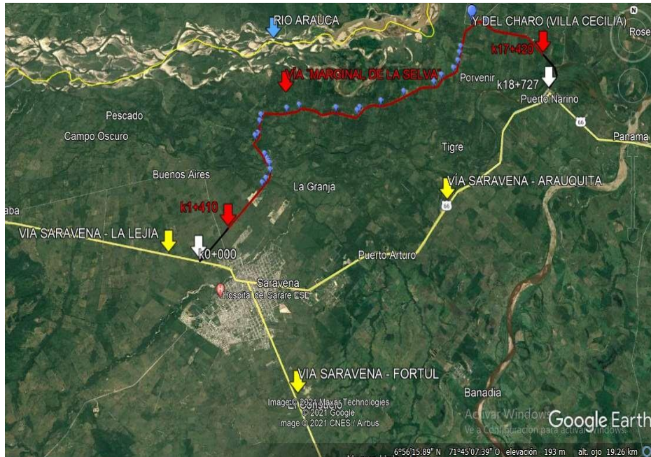
Figura 3. Implantación General del Proyecto
