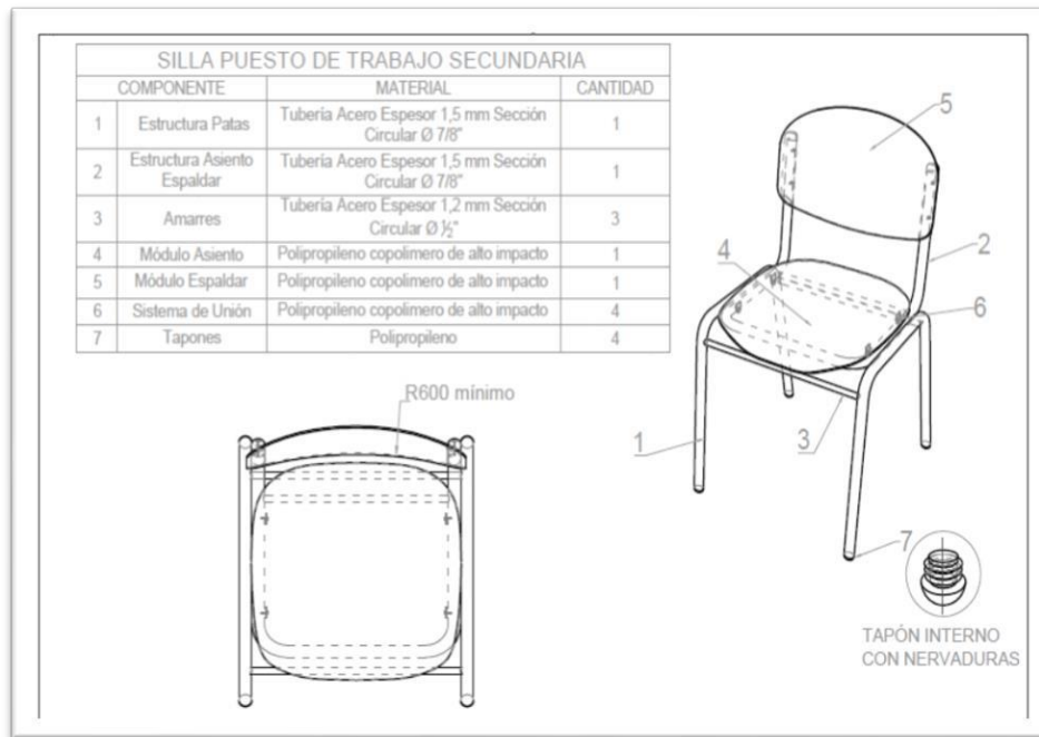
Ilustración 7 Silla Puesto de Trabajo Secundaria
