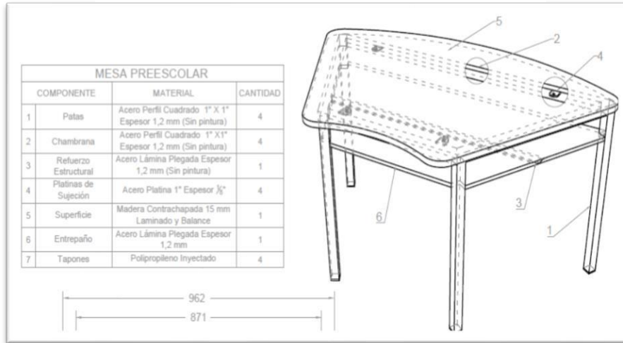
Ilustración 4 Mesa Puesto de Trabajo Preescolar
