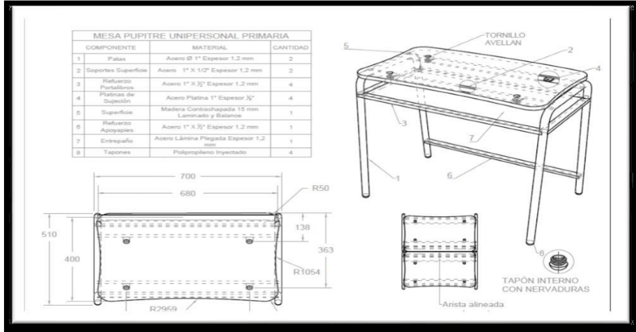
Ilustración 5 Mesa Puesto de Trabajo Primaria
