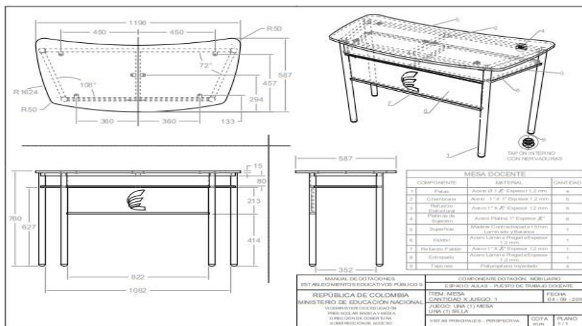
Ilustración 10 Mesa Puesto de Trabajo Docente
