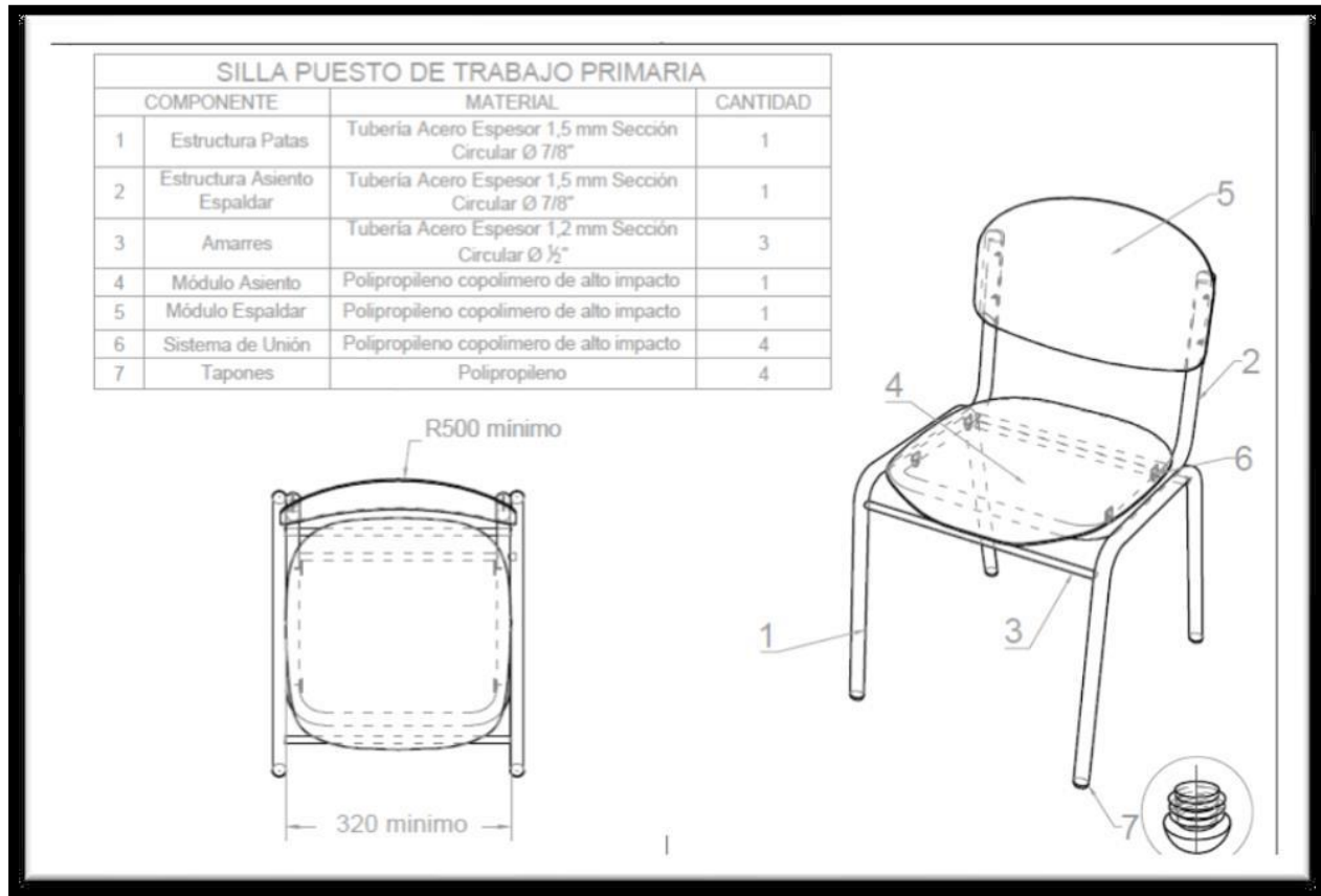
Ilustración 6 Silla Puesto de Trabajo Primaria
