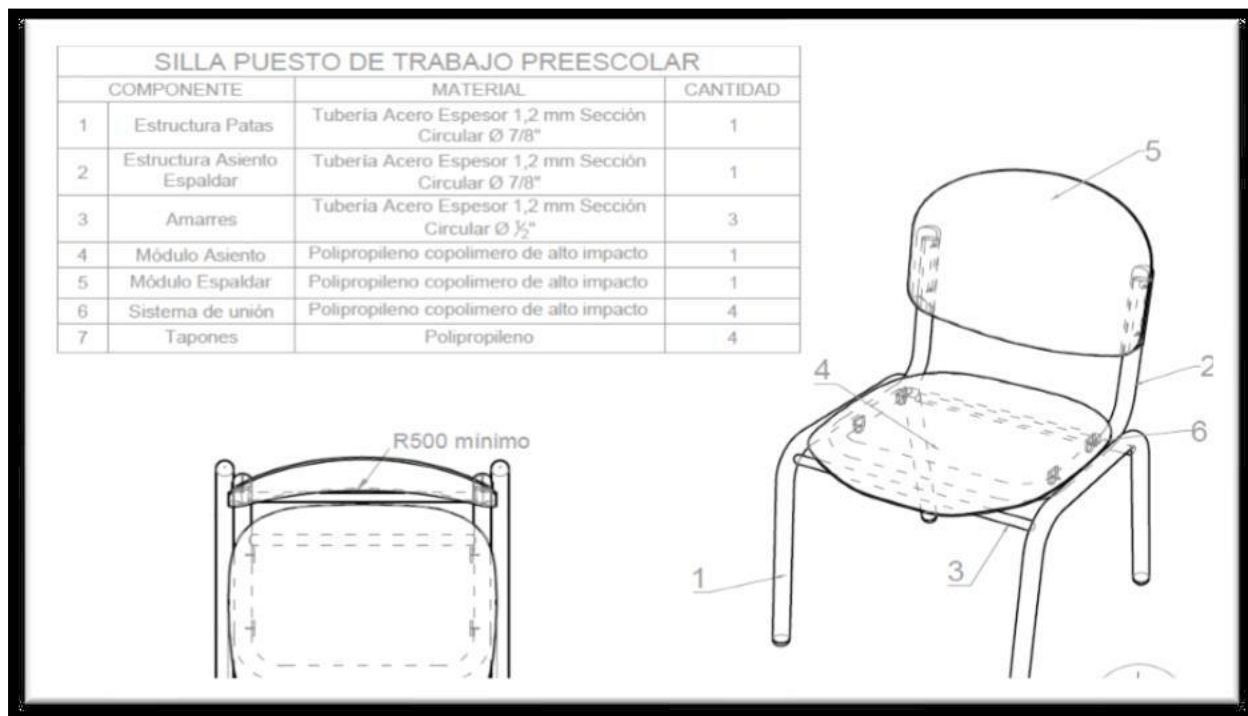
Ilustración 3 Silla Puesto de Trabajo Preescolar
